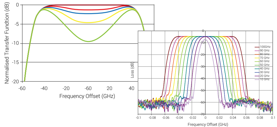
Mux/DeMux
